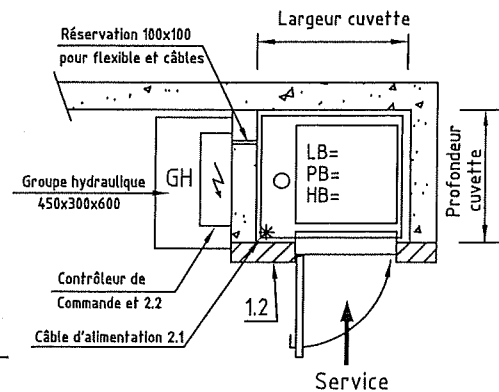
VUE EN PLAN AU: S/S
