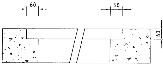
DETAIL FEUILLURE
